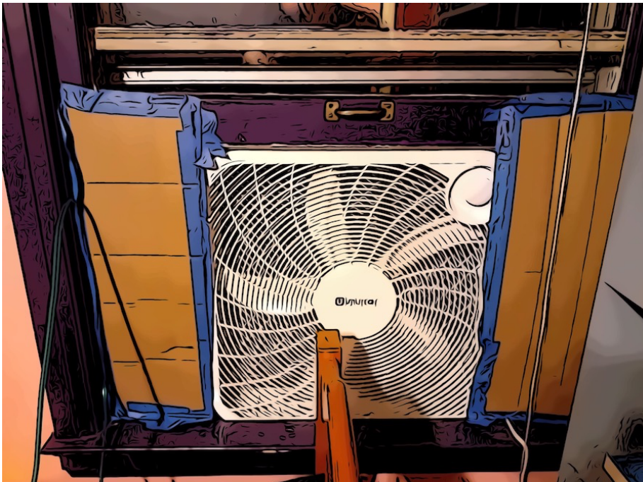
Foto 3. Ventilador de caja montado en la ventana para soplar el aire del exterior dentro la habitación, sellado a los lados.
